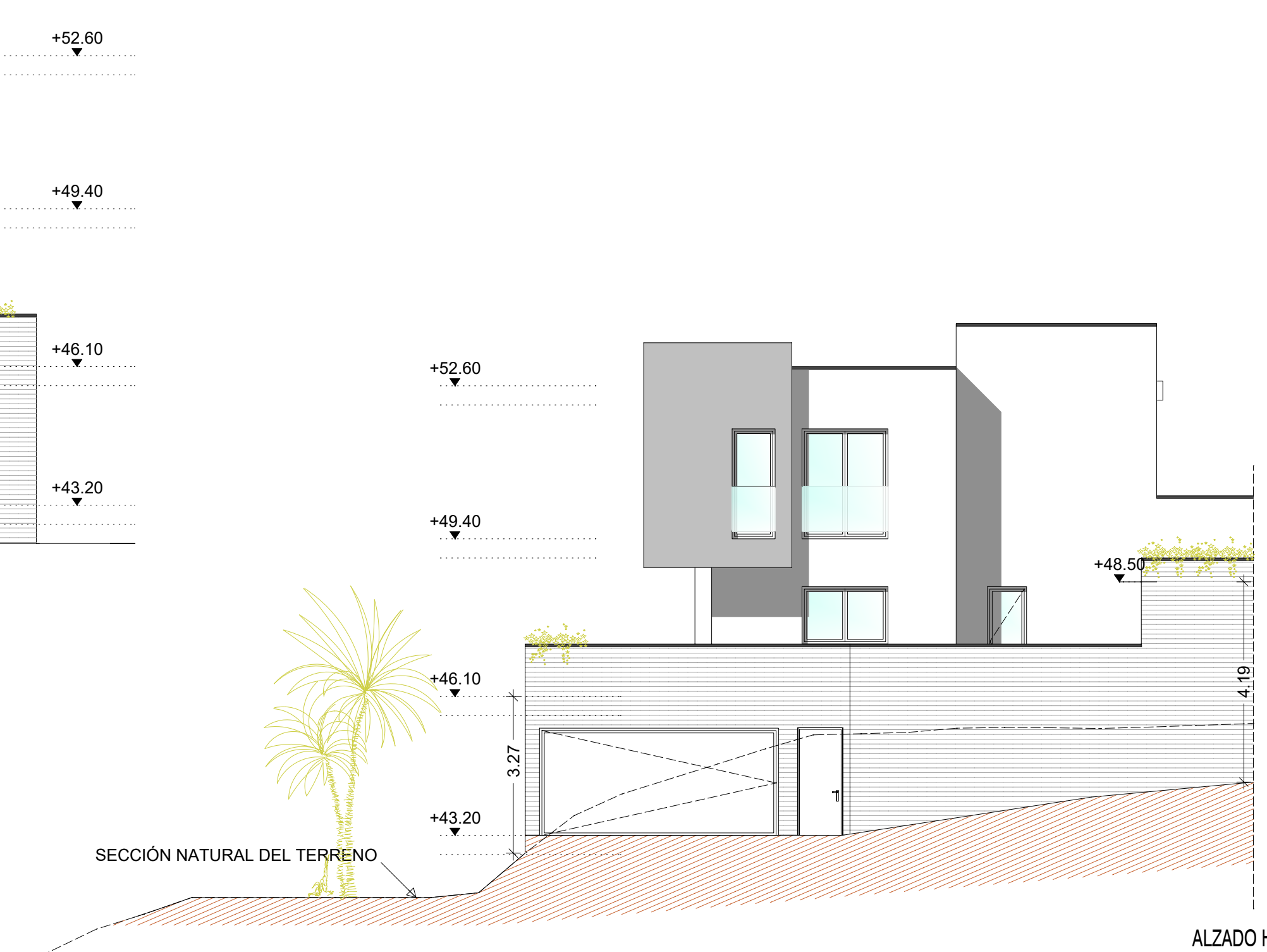
ALZADO I
