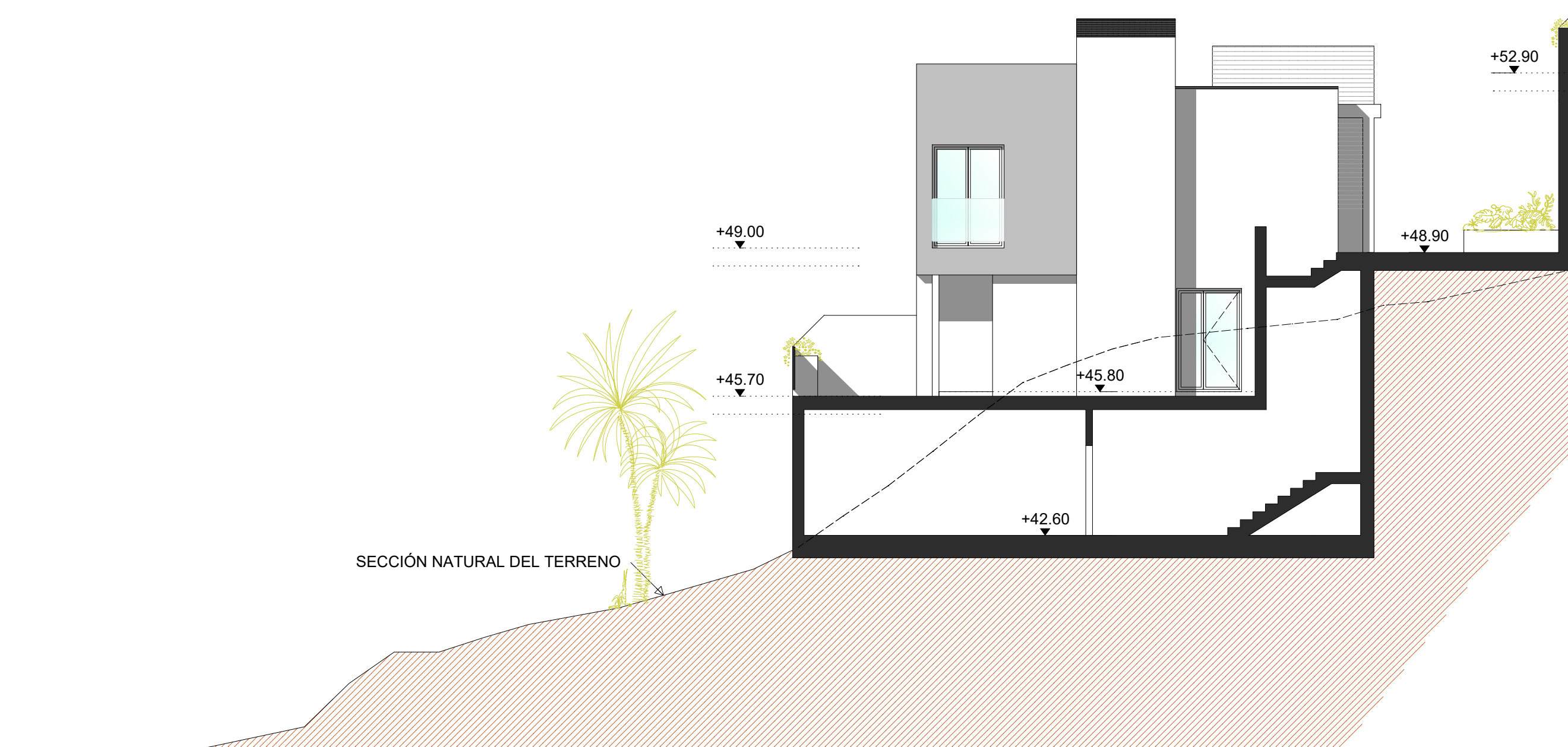
ALZADO H
